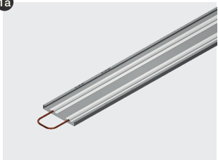
Heat Panel for afslutning Mål: 3000 (2700) x 297 x 30 mm Materiale: Aluminium med kobberregister Vægt: 1,37 kg/stk.
