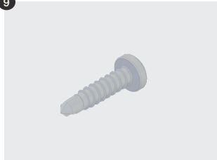
Selvskærende skruer Mål: ø 4,1 x 13 mm Materiale: Stål
