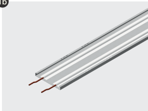
Heat Panel, standard Mål: 3000 (2700) x 297 x 30 mm Materiale: Aluminium med kobberregister Vægt: 1,37 kg/stk.
