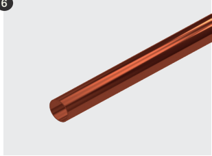
Kobberrør Mål: ø 12 x 116 mm Materiale: Kobber Vægt: 125 g/stk.
