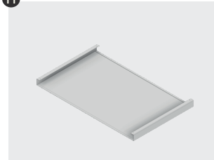
Dækplade* Mål: 372 x 600 x 35 mm Materiale: Aluminium Vægt: 760 g/stk.
