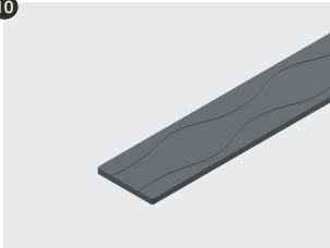
Batts i pose Mål: 1200 x 295 mm Materiale: Mineraluld i pose Vægt: 440 g/stk.
