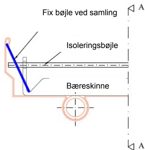
Sektion A-A
