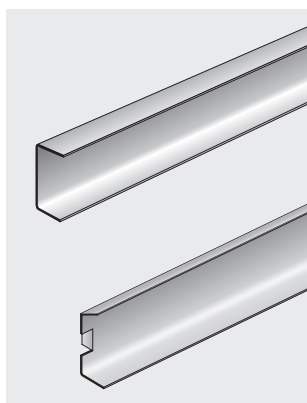
Kantliste nr. 36 Kan leveres konkav eller konveks Mål: 15 × 38 × 15 × 4000 mm Materiale: Galvaniseret stål Overflade: Lakeret
