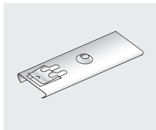
Bæreskinnelaske nr. 4 Mål: 12 × 40 × 110 mm Materiale: Galvaniseret stål
