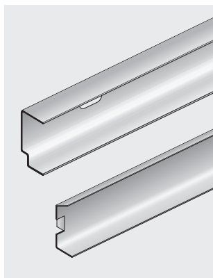
Skyggekantliste nr. 6 Kan leveres konkav eller konveks Mål: 20 × 38 × 14 × 4000 mm Skygge: 6 × 9 mm Materiale: Galvaniseret stål Overflade: Lakeret
