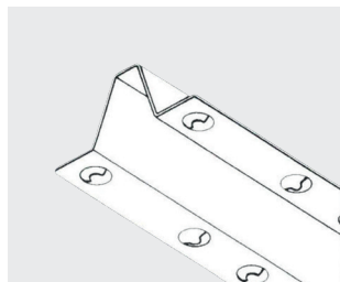
Modulbæreskinne til DAMPA® Sport Mål: 35 × 87 × 4000 mm Materiale: Galvaniseret stål
