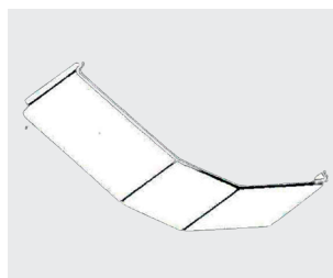
Låseclips nr. 5 Mål: 23 × 87 × 1,5 mm Materiale: Galvaniseret stål Overflade: sortlakeret
