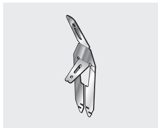
Stroplås nr. 5 Mål: 26 × 40 × 175 mm Materiale: Galvaniseret fjederstål
