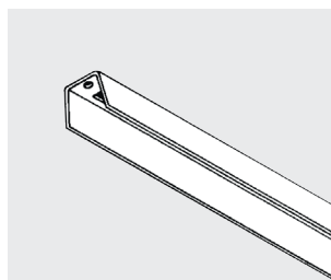
Bæreskinnelaske til DAMPA® Sport Mål: 28 × 21 × 300 mm Materiale: Galvaniseret stål
